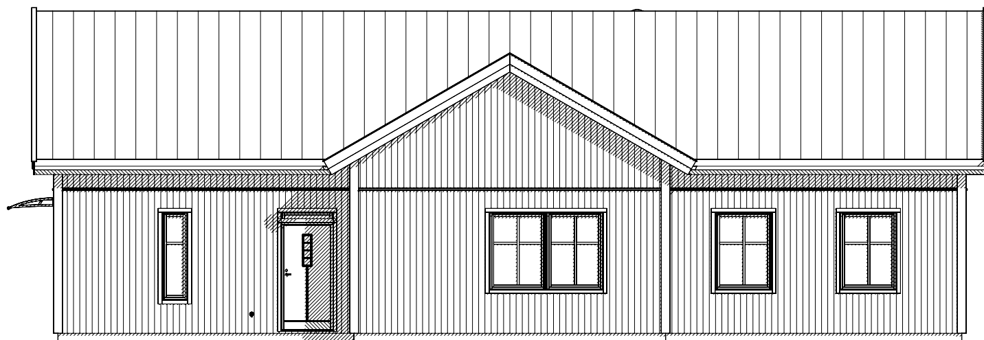
FASAD MOT SYDÖST
